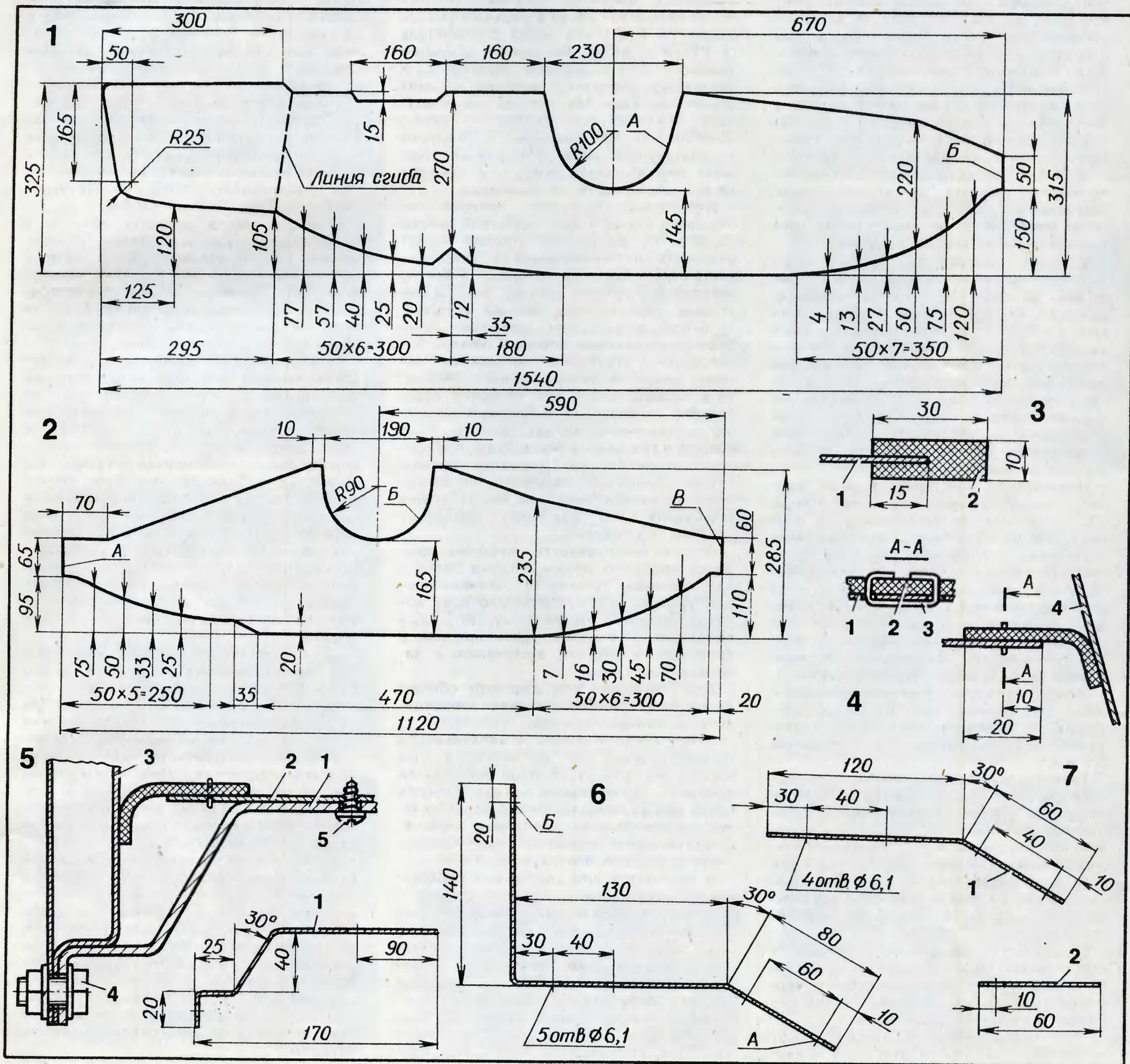
Рис. 7. Детали крепления заднего щитка: 1 — кронштейн; 2 — планка.
